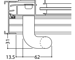
樹脂製把手 (標準装備外)
