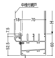
※ガラス溝幅 14mm 下枠外部アタッチ (18mm) を取付ける場合
