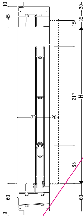
大型下框 (標準装備)
