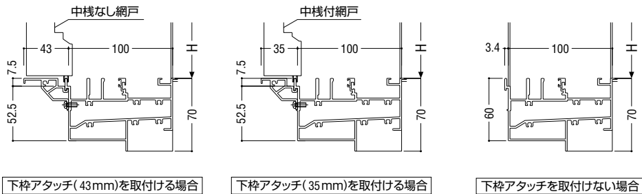
下枠アタッチ(43mm)を取付ける場合
