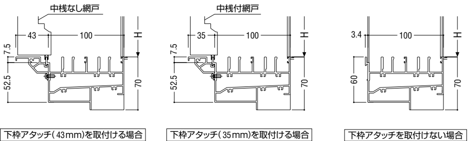
下枠アタッチ(43mm)を取付ける場合
