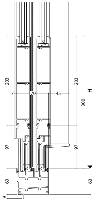
大型下枠 (標準装備外)
