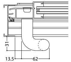
樹脂製把手 (標準装備外)
