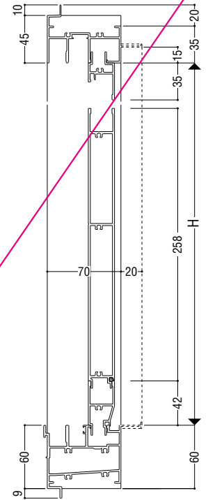
大型下框 (標準装備)
