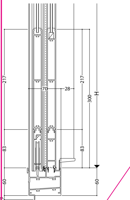
大型下框 (標準装備外) FIX部15mm
