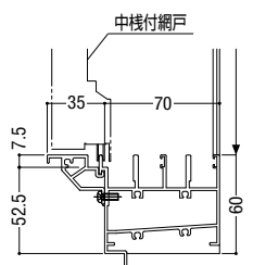
※ガラス溝幅 14mm 下枠外部アタッチ (35mm) を取付ける場合
