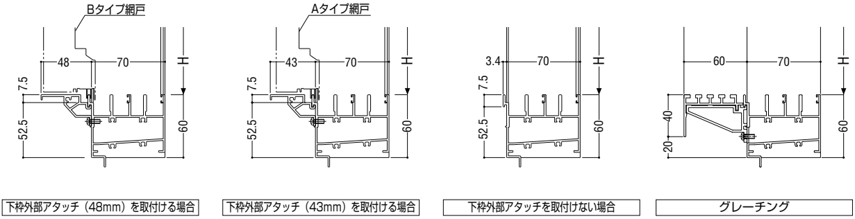
下枠外部アタッチ (48mm) を取付ける場合
