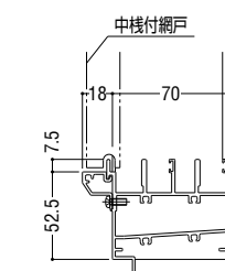
※ガラス溝幅 14mm 下枠外部アタッチ (18mm) を取付ける場合
