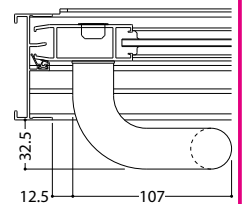
ステンレス製把手 (標準装備外)
