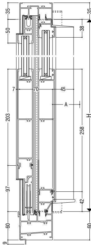
大型下框 (標準装備)
