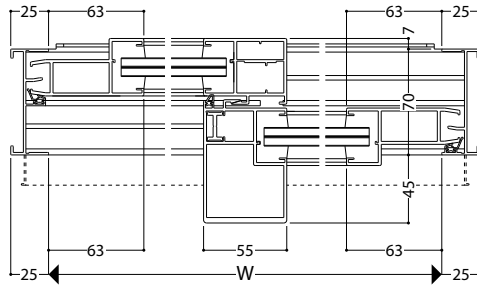
ガラス溝幅28mm
