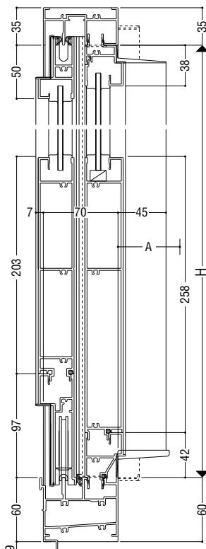
大型下枠 (標準装備)
