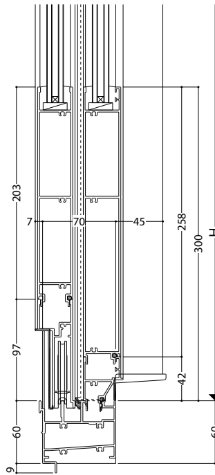
大型下框 (標準装備外)
