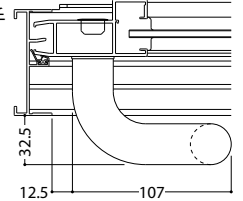
ステンレス製把手 (標準装備外)
