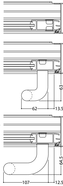
ガラス溝幅14mm
