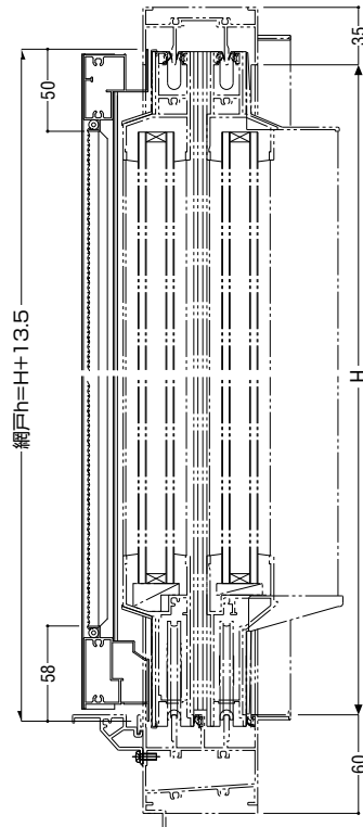
引違い(A・Bタイプ)
