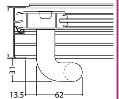
樹脂製把手 (標準装備外)
