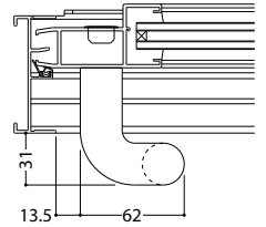
樹脂製把手 (標準装備外)
