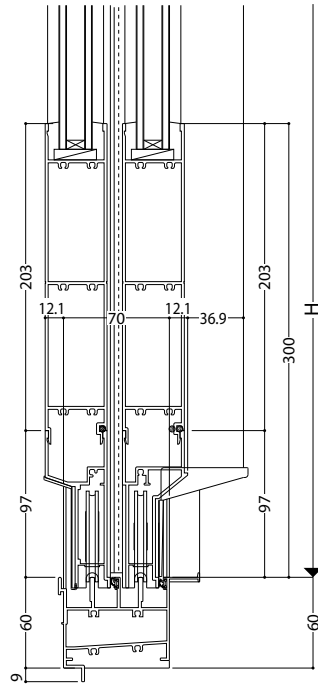
大型下枠 (標準装備外)
