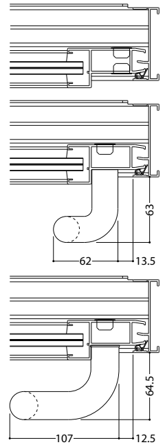
ガラス溝幅28mm
