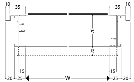
ガラス溝幅14mm
