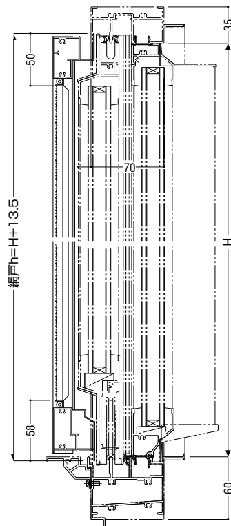
外動片引き(A・Bタイプ)
