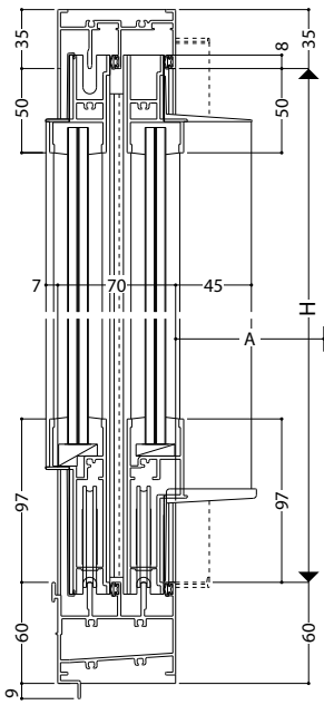
大型下枠 (標準装備外) ガラス溝幅14mm
