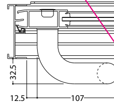
ステンレス製把手 (標準装備外)
