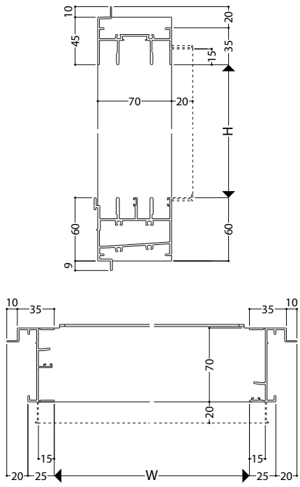
大型下枠 (標準装備外)
