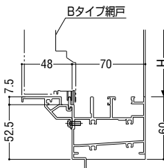
下枠外部アタッチ (48mm) を取付ける場合
