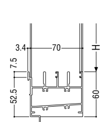
下枠外部アタッチを取付けない場合
