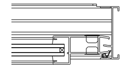
彫り込み引手 (標準装備)
