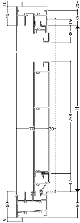
大型下框 (標準装備)
