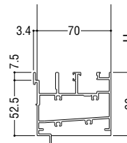
下枠外部アタッチを取付けない場合
