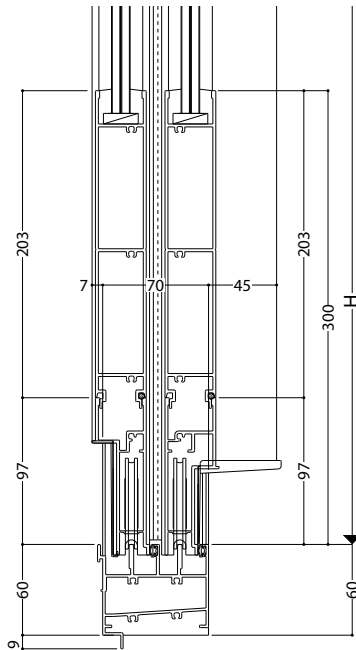
ガラス溝幅28mm
