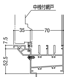
※ガラス溝幅 14mm 下枠外部アタッチ (35mm) を取付ける場合
