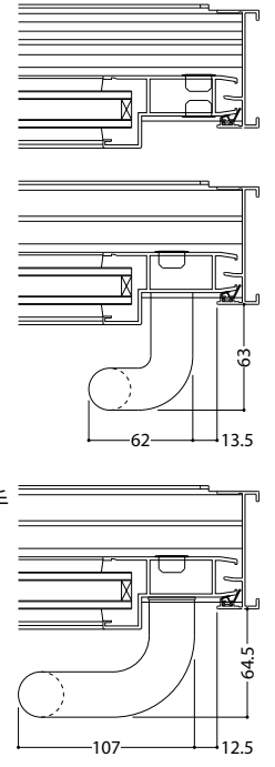
ステンレス製把手 (標準装備外)
