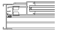
彫り込み引手 (標準装備)
