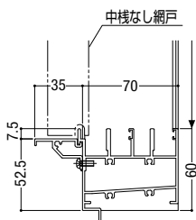
※ガラス溝幅 14mm 下枠外部アタッチ (35mm) を取付ける場合
