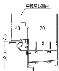
下枠外部アタッチ (43mm) を取付ける場合
