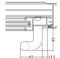
樹脂製把手 (標準装備外)
