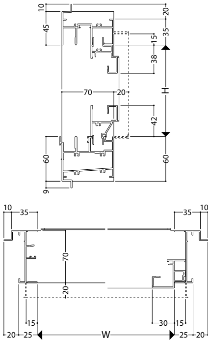
大型下框 (標準装備外)
